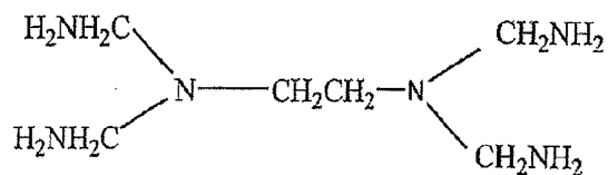
EDTA
