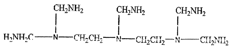
DTPA
